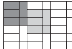
Vzorec polaganja št. 5
