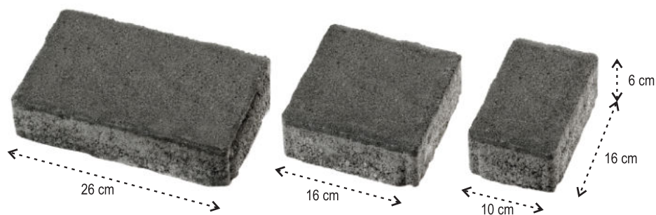
Vzorec polaganja št. 3
