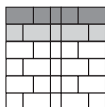
Verlegemuster Nummer 2
