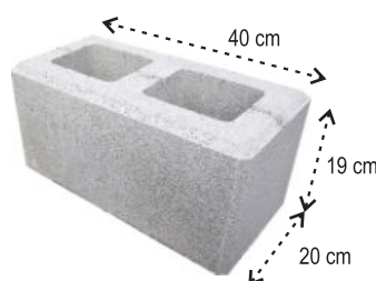
NORMALSTEIN GLATT
